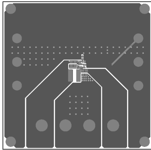
Figure 4—Top Layer
