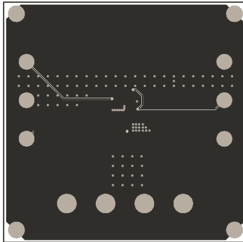
Figure 5—Bottom Layer
