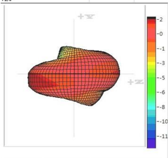
600MHzRight-Left View
