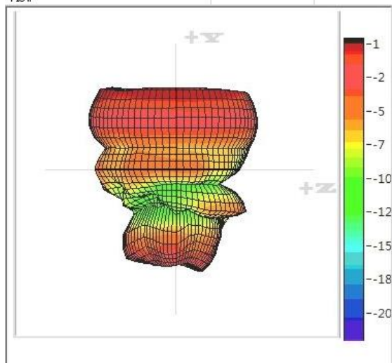
4.8GHzRight-Left View
